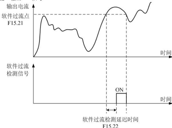
图 5-29 软件过流检测示意图
