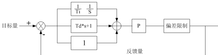
图 5-24 过程 PID 原理框图
