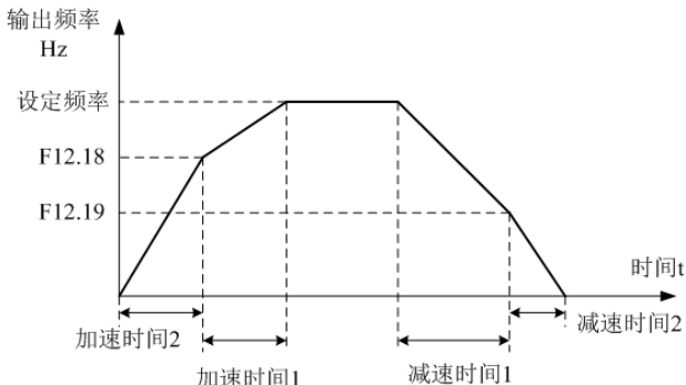
图 5-22 加减速时间切换示意图
