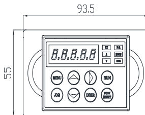
八键键盘外形尺寸
