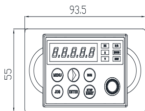
六键键盘外形尺寸
