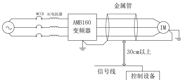
图 3-8 传导干扰对策
