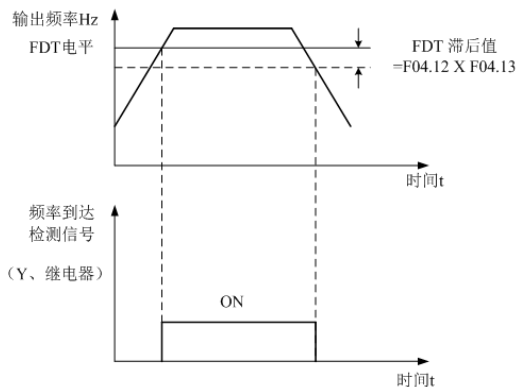
图 5-8 FDT 电平示意图
