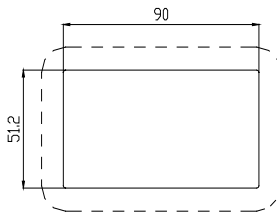
外引键盘(六键、八键)开孔尺寸图
