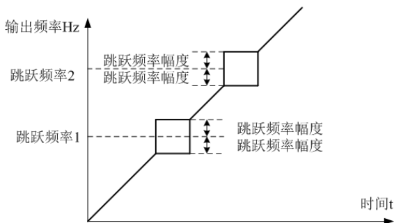
图5-20 跳跃频率示意图
