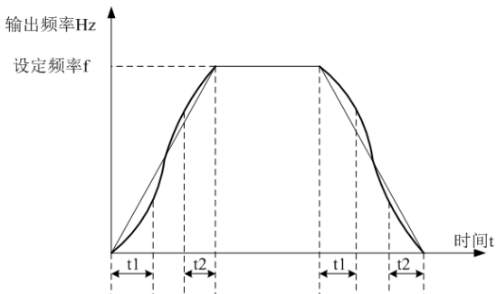
图 5-12 S 曲线加减速 A 示意图
