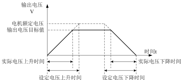
图 5-18 V/F 分离示意图
