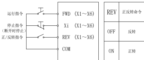
图 5-6 3 线制顺序控制模式 2
