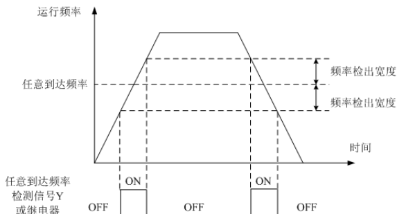
图 5-10 任意到达频率检测示意图
