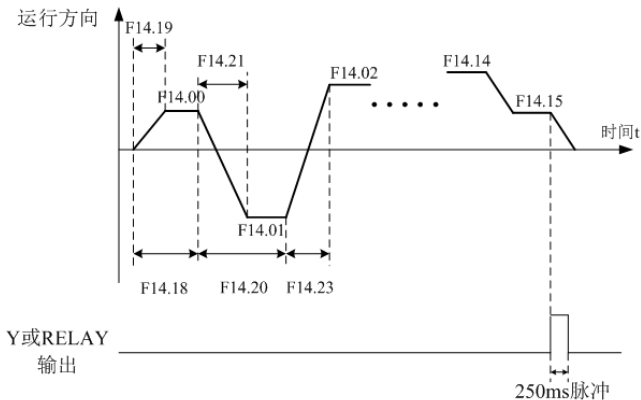
图 5-27 简易 PLC 示意图
