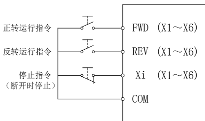
图 5-5 3 线制顺序控制模式 1
