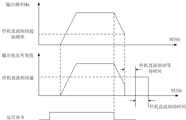
图 5-14 停机直流制动示意图
