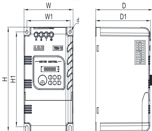
7.5KW 规格外型尺寸
