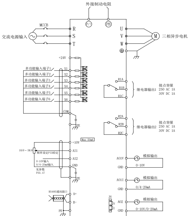
图 3-13 控制回路端子连接图
