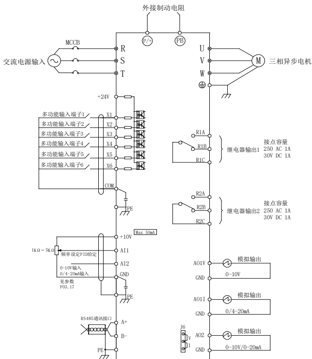
图 3-2 AMB160 变频器连接图
