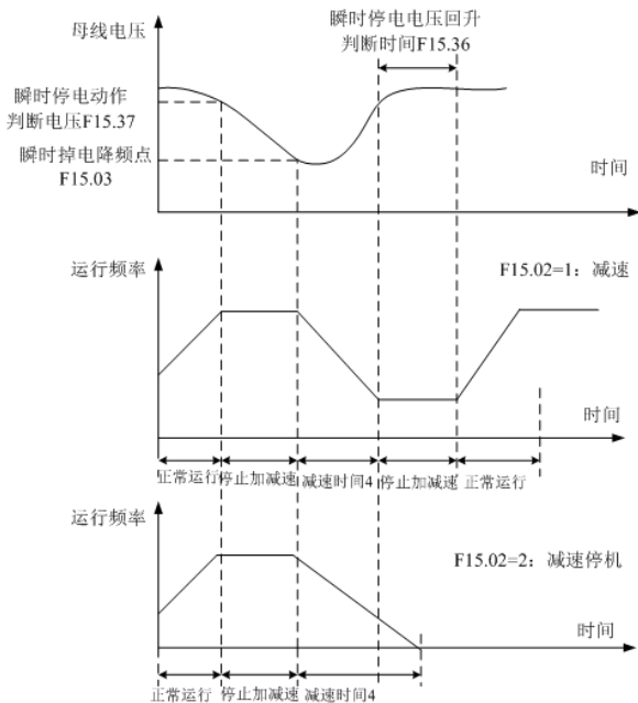
图 5-28 瞬时掉电动作示意图
