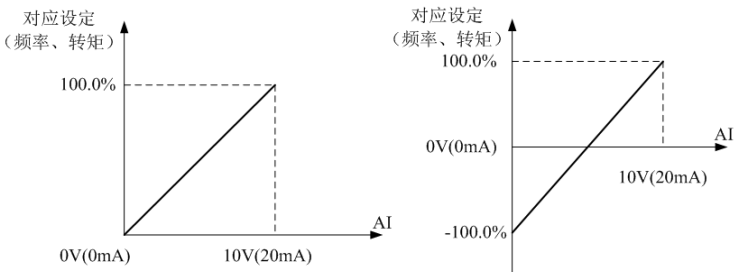
图 5-7 模拟给定与设定量的对应关系
