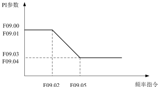
图 5-19 PI 参数示意图
