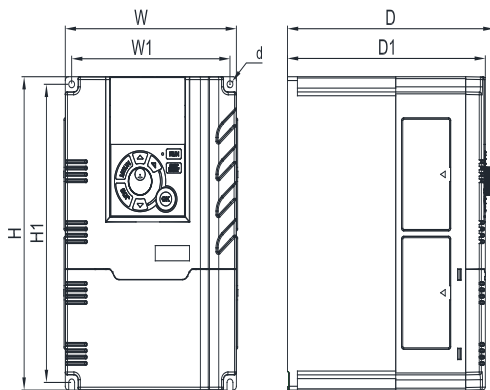
11KW 规格外型尺寸
