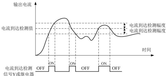
图 5-11 电流到达检测示意图
