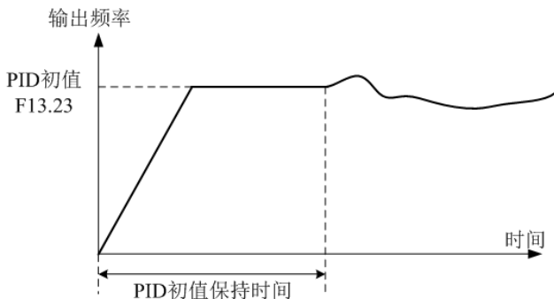
图 5-26 PID 初值功能示意图
