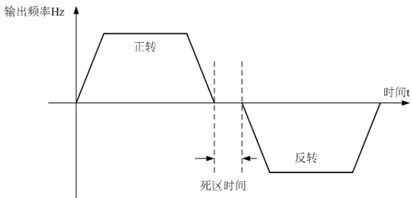
图 5-15 正反转死区时间示意图
