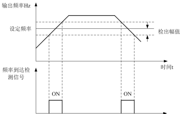
图 5-9 频率到达检出幅值示意图
