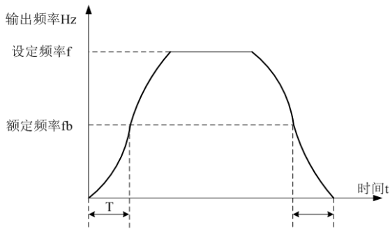
图 5-13 S 曲线加减速 B 示意图
