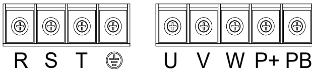
三相 380V(0.75-2.2KW)主回路端子 图 1-2 控制回路端子和主回路端子配置
