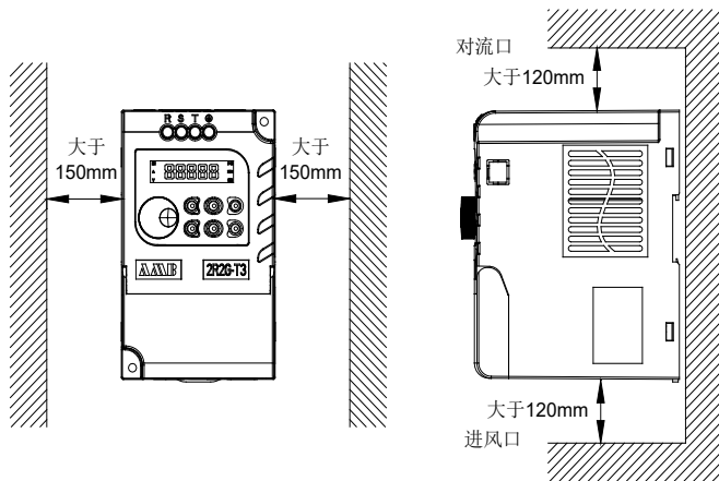
图 2-2 AMB160 变频器安装方向和空间
